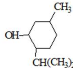
2-Isopropyl-5-methylhexanol
