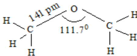
Methoxyethane
