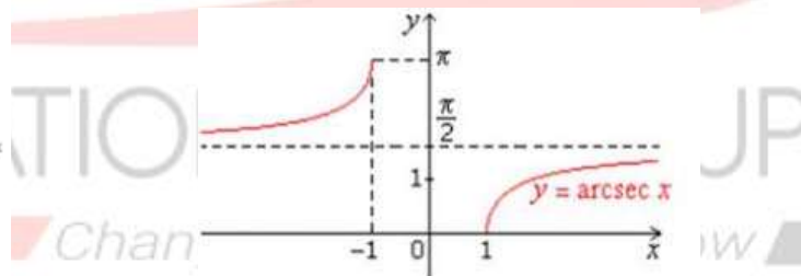
y = \sec^{-1} x
