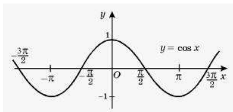
y = \cos x
