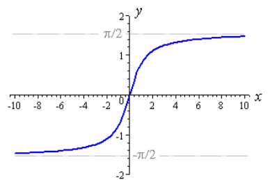
y = \tan^{-1} x
