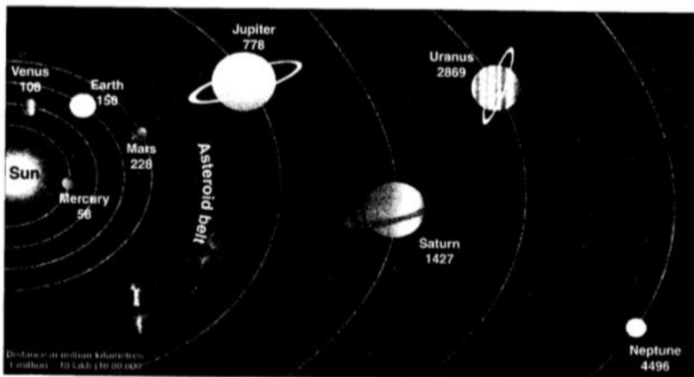
Fig. 1.4. Solar System.
